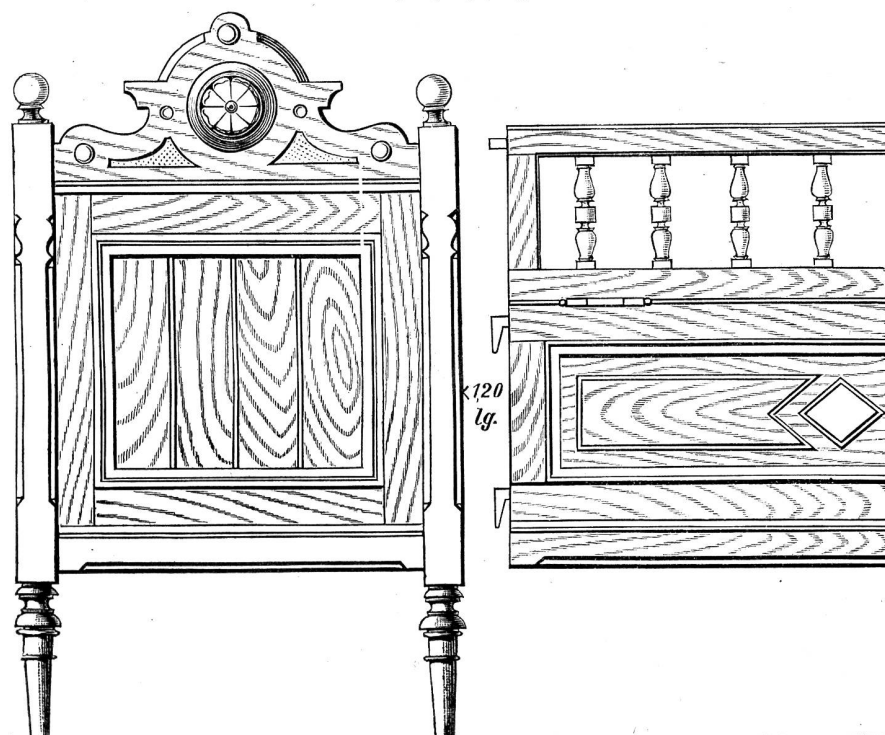
Kinderbettstelle.
