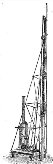
Rammarbeiten. [380 (M 10226 Z)] Besteingerichtete Gerüste auf Dielenunterlagen, Geleisen und Pontons.
