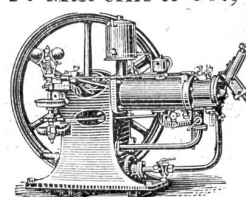
Fräs-Maschine.
