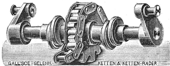
GALL'SCHE GELENK-KETTEN-UND KETTEN-RÄDER
