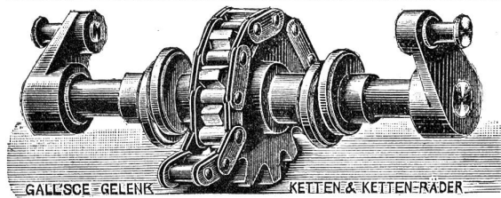
GALL'SCE-GELENK KETTEN-&KETTEN-RÄDER
