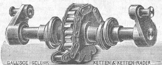
GALL'SCHE GELENK
