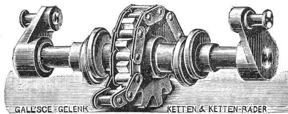
GALL'SCHE GELENK KETTEN & KETTEN-RÄDER
