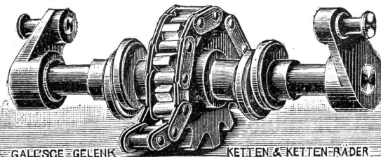
GALL'SCHE GELENK KETTEN- u. KETTEN-RÄDER
