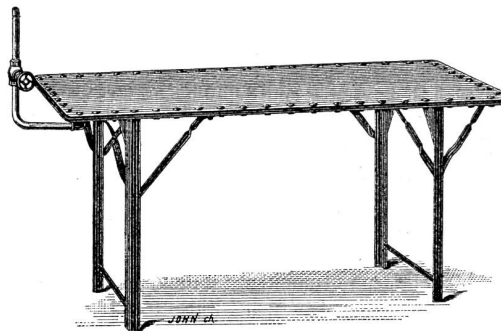
Nr. 2. Dampfleimtisch.
