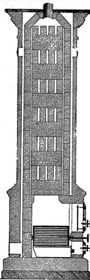
PATENT-OFEN MIT SUTER-EINBAU. QUERSCHNITT. POLLE SUTER, BREVETÉ (S. O. D. O.) SUOIS. TRANSMISSION.
