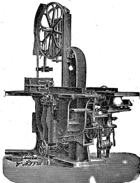
Universalmaschine solidester Konstruktion.
