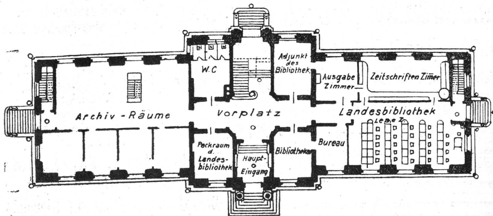
Grundriß.
