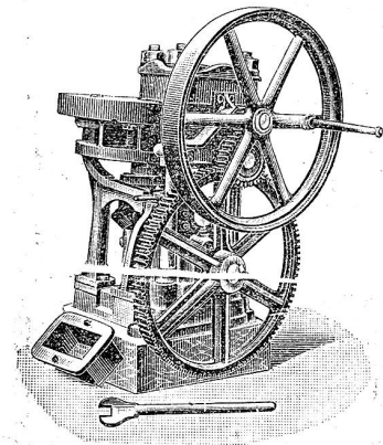
Excenterpresse
