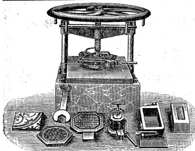
Spindelpresse
