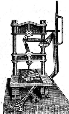
Kniehebelpresse
