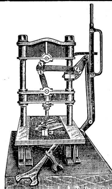
Kniehebelpresse
