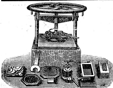
Spindelpresse
