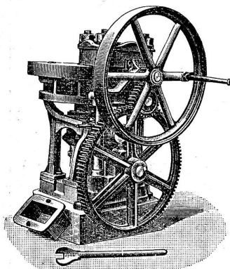
Excenterpresse
