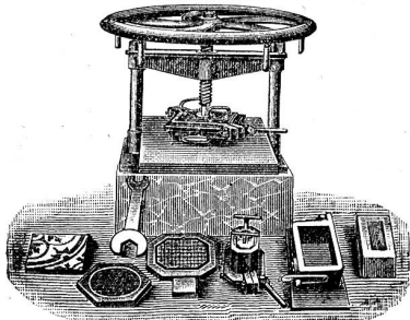
Spindelpresse
