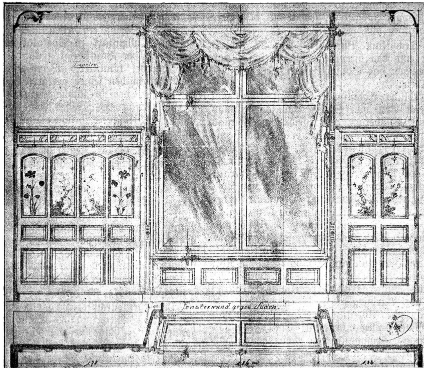
C. Fensterwand. Entworfen von A. Schirich, Atelier für Bau- und Möbelzeichnungen, Zürich I. Ausgeführt von Theoph. Ginnen, mech. Bauschreinerei, Zürich V.
