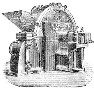
Universalmühle
