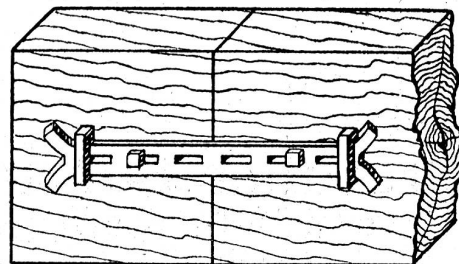
Verbindungsschiene.
