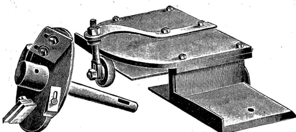
Abplattkopf mit Schutzvorrichtung
