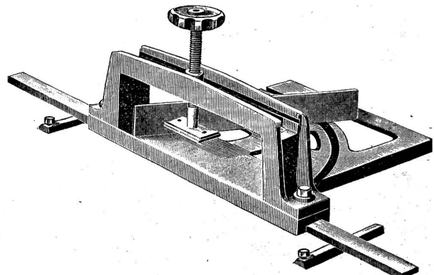
Zapfenschneidtischchen
