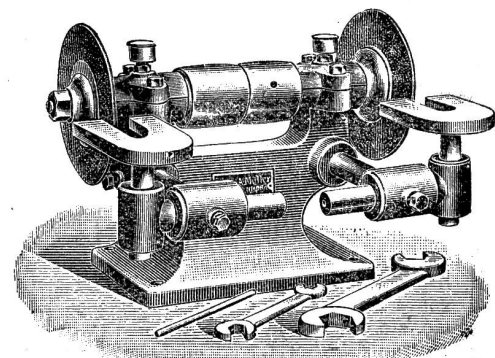
Kehlmesserschleifapparat
