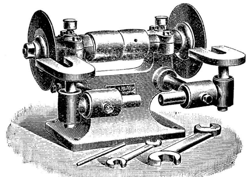
Kehmesserschleifapparat
