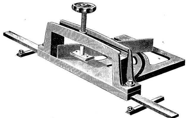
Zapfenschneidtischchen
