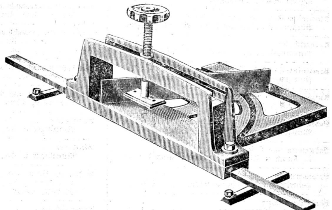
Zapfenschneidmaschine
