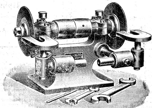
Kehlmesserschleifapparat
