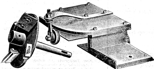
Abplattkopf mit Schutzvorrichtung
