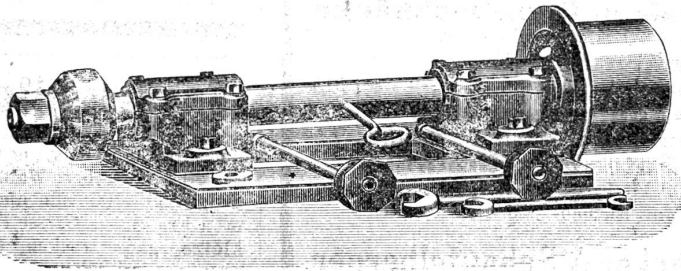
Kreissägenwelle
