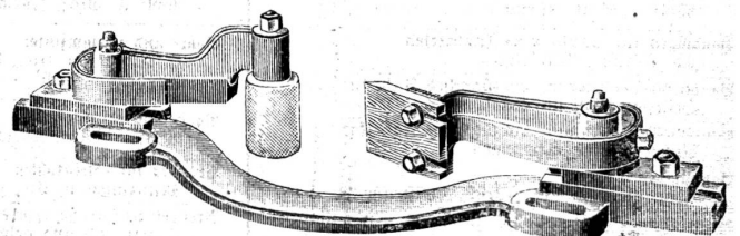
Kehlranddruckapparat
