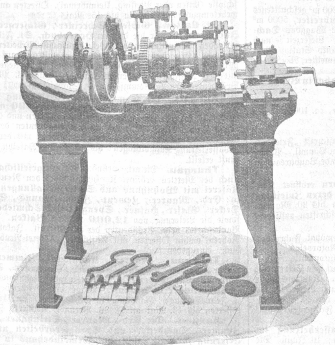
Fräser-Hinter-Drehbank.
