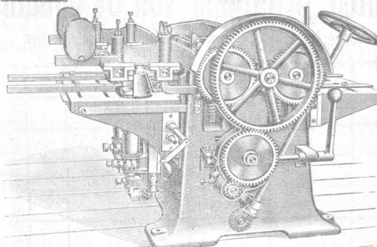
Dreiseitige Hobelmaschine.
