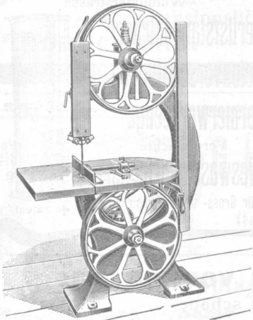
Kleinere Bandsäge.
