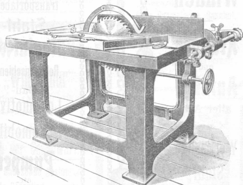
Kreissäge
