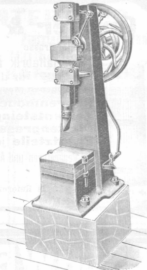
Holzspaltmaschine.
