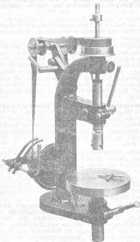
Schnellbohrmaschine „EXAKT“, Preis Fr. 98.
