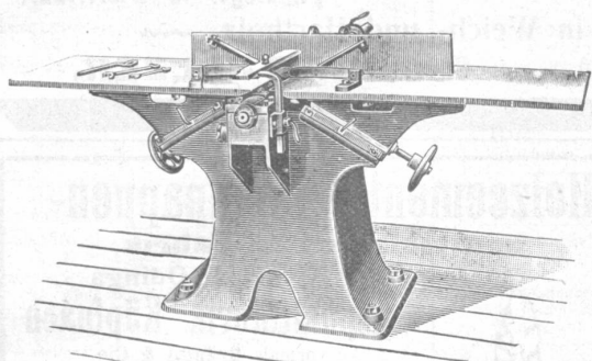
Abrichtmaschine.
