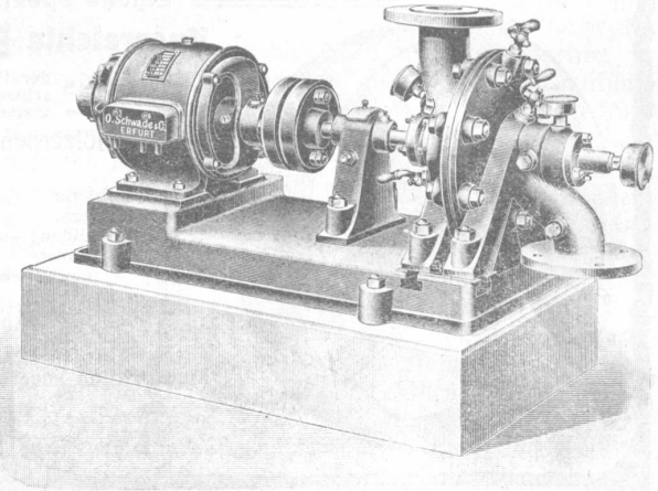
Fig. 15. Einstufige Hochdruck-Zentrifugalpumpe. (Elektromotor-Antrieb.)
