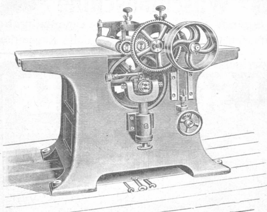
Sandpapierschleifmaschine.
