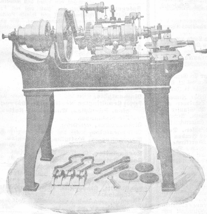
Fräser-Hinter-Drehbank.
