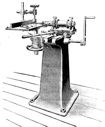
Langlochbohrmaschine.
