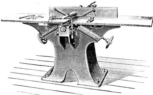
Abrichtmaschine.
