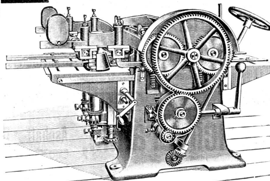
Dreiseitige Hobelmaschine.
