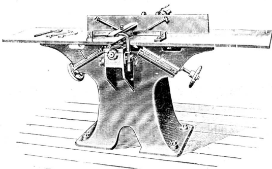
Abrichtmaschine.
