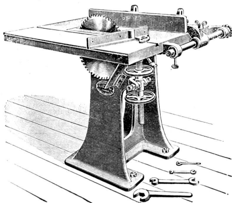
Kreissäge
