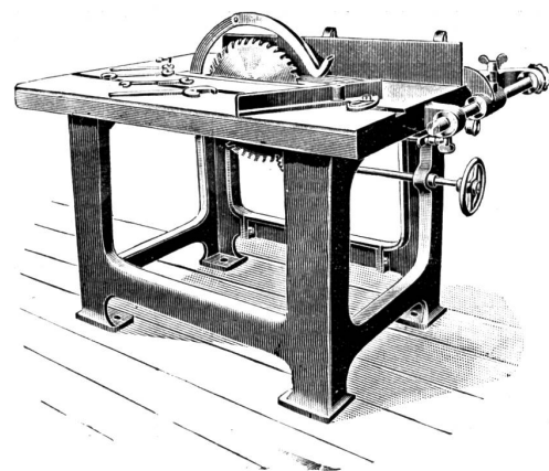
Kreissäge
