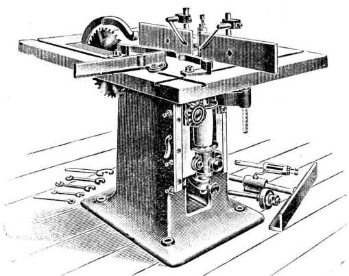
Kreissäge kombiniert mit Kehlmaschine.
