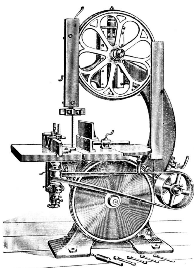
Bandsäge kombiniert mit Kehlmaschine.
