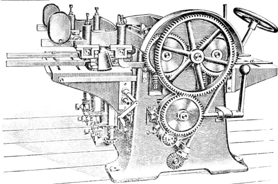
Dreiseitige Hobelmaschine.
