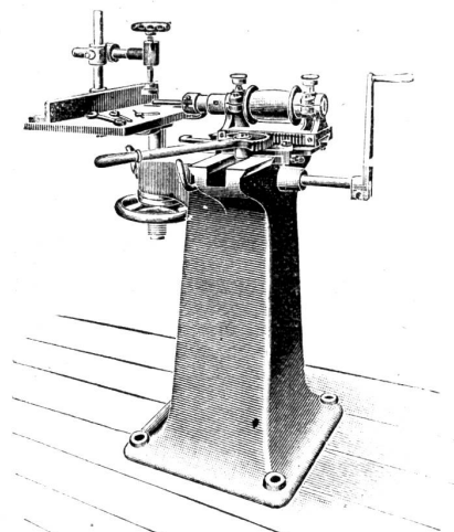
Langlochbohrmaschine.
