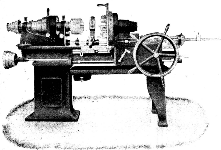
Revolver-Drehbank R 35.
