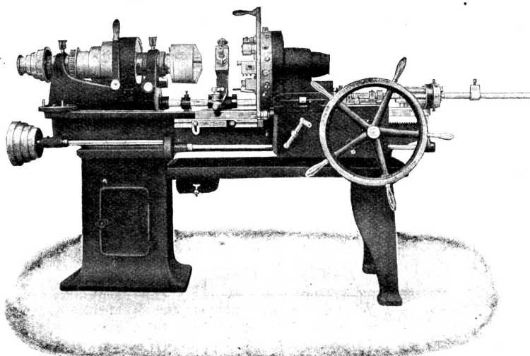
Revolvier-Drehbank R 35.
