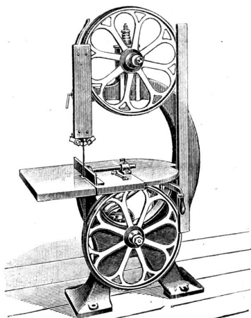
Kleinere Bandsäge.
