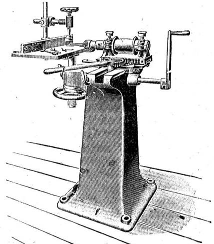
Langlochbohrmaschine.
