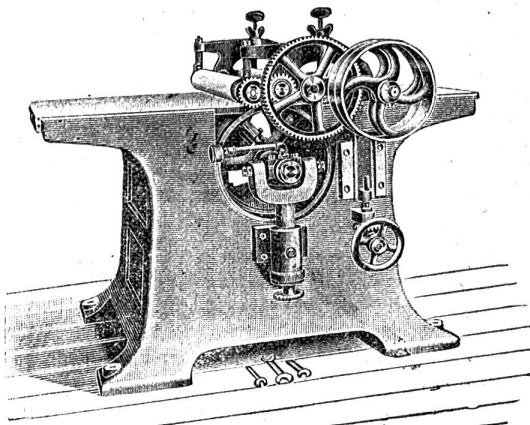
Sandpapierschleifmaschine.
