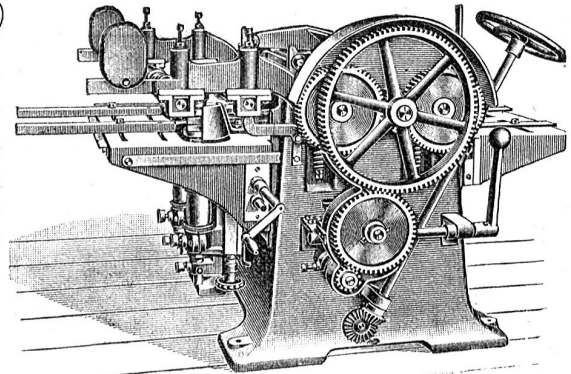
Dreiseitige Hobelmaschine.
