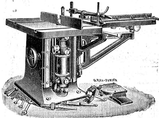
Kombinierte Kehl- und Zapfenschneidmaschine.
