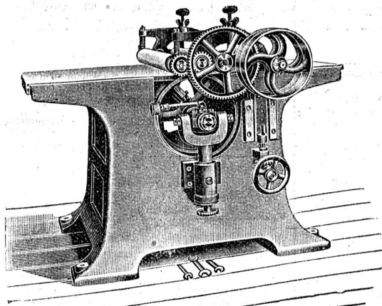
Sandpapierschleifmaschine.
