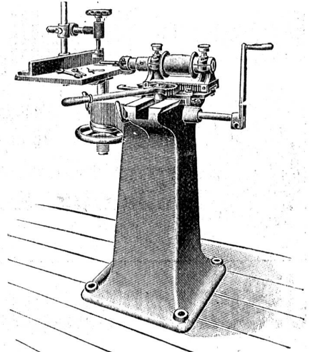
Langlochbohrmaschine.
