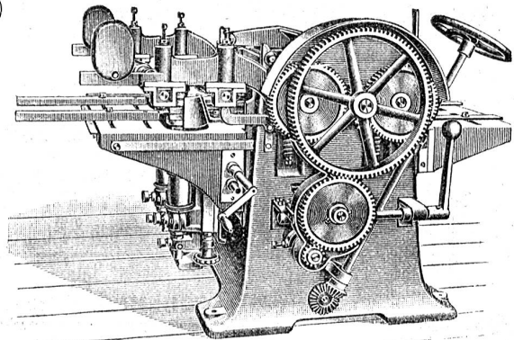
Dreiseitige Hobelmaschine.
