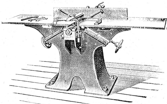
Abrichtmaschine.
