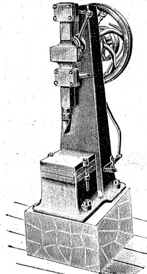
Holzspaltmaschine.
