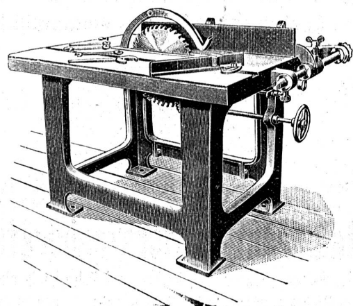
Kreissäge
