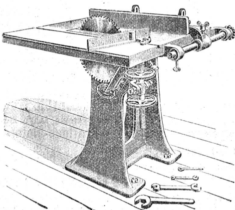
Kreissäge
