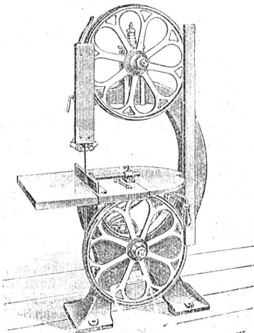
Kleinere Bandsäge.
