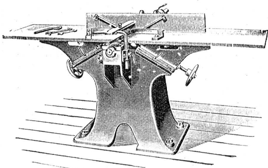
Abrichtmaschine.
