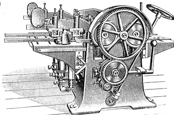
Dreiseitige Hobelmaschine.
