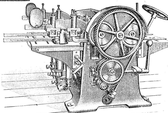
Dreiseitige Hboelmaschine.
