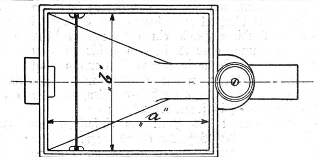
Fig. 3. Draufsicht.
