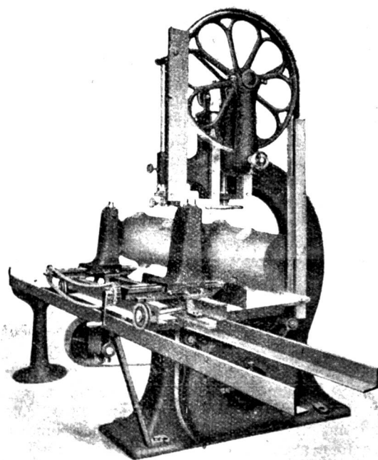
Bandsäge mit Laufwagen mit selbsttätigem Vorschub.
